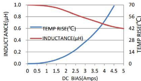
PML2010-1R0-N
